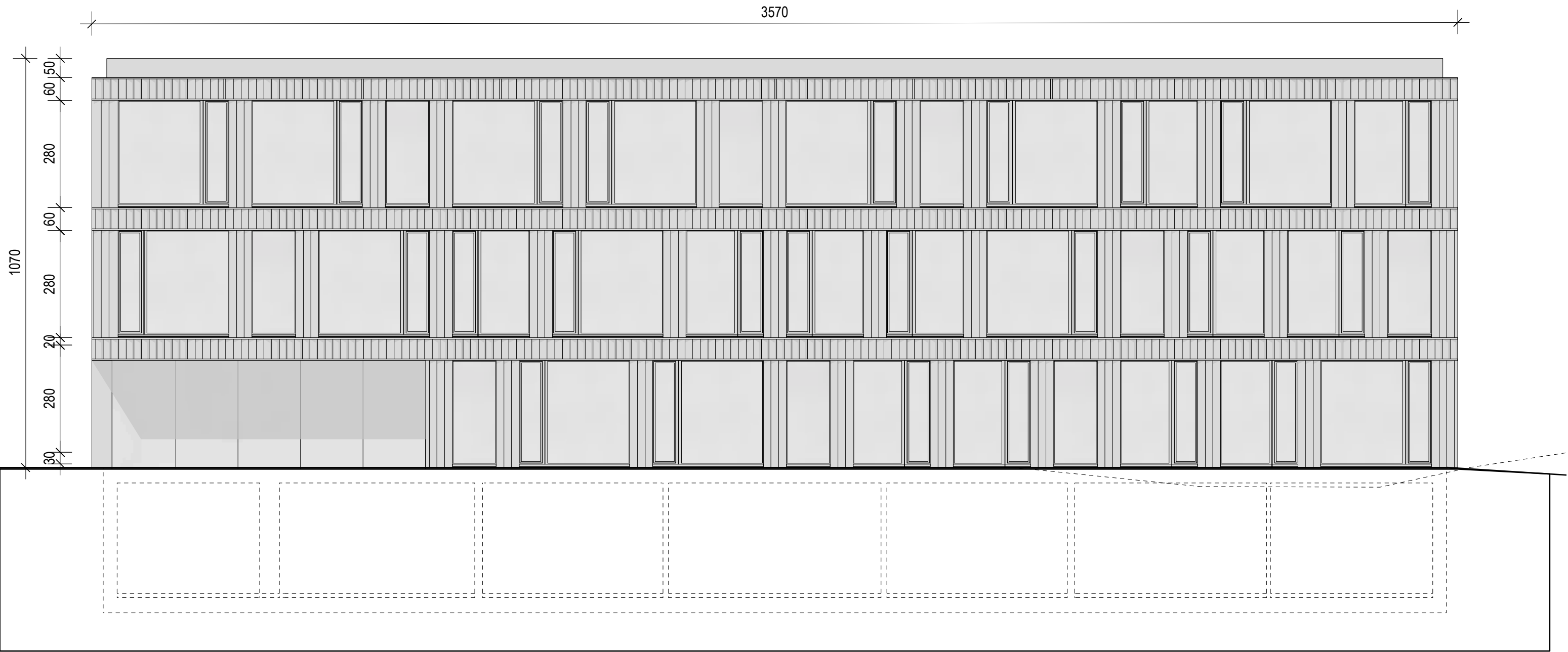
FAÇADE NORD-EST
