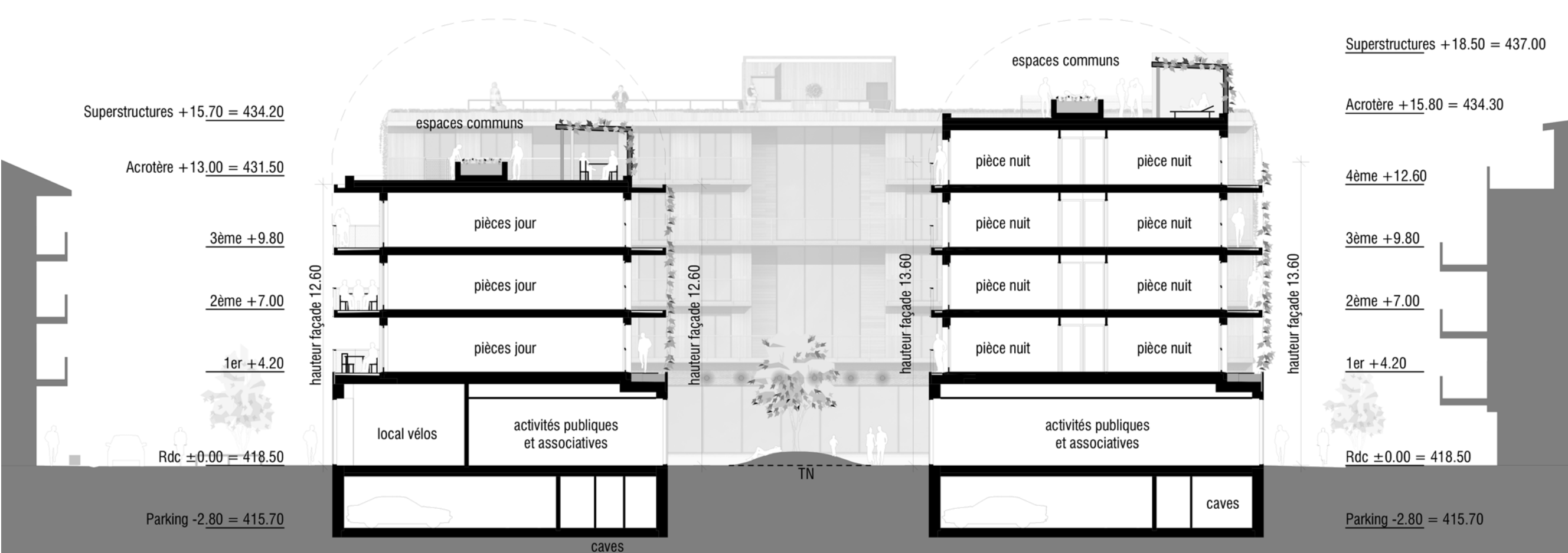
Coupe longitudinale AA Ech : 1/200°
